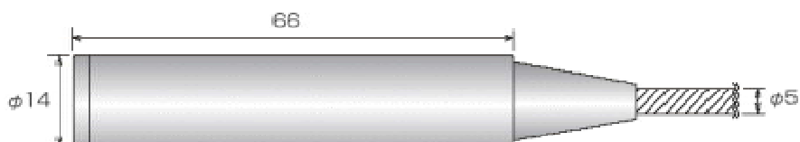
WML-N1W 外形寸法 WML-N1A
